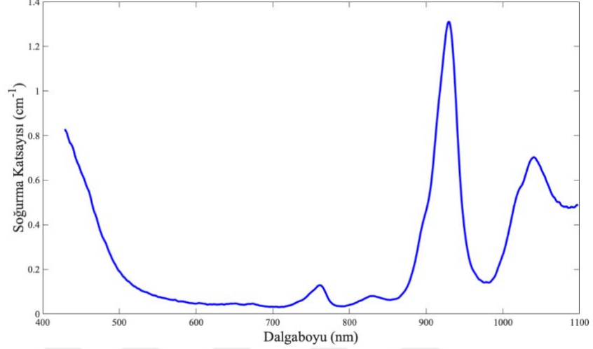
Şekil 2.6 Lipitlerin 450 - 1100 nm aralığında dalga boyuna bağlı olarak soğurma katsayısı (Van, 2004)
